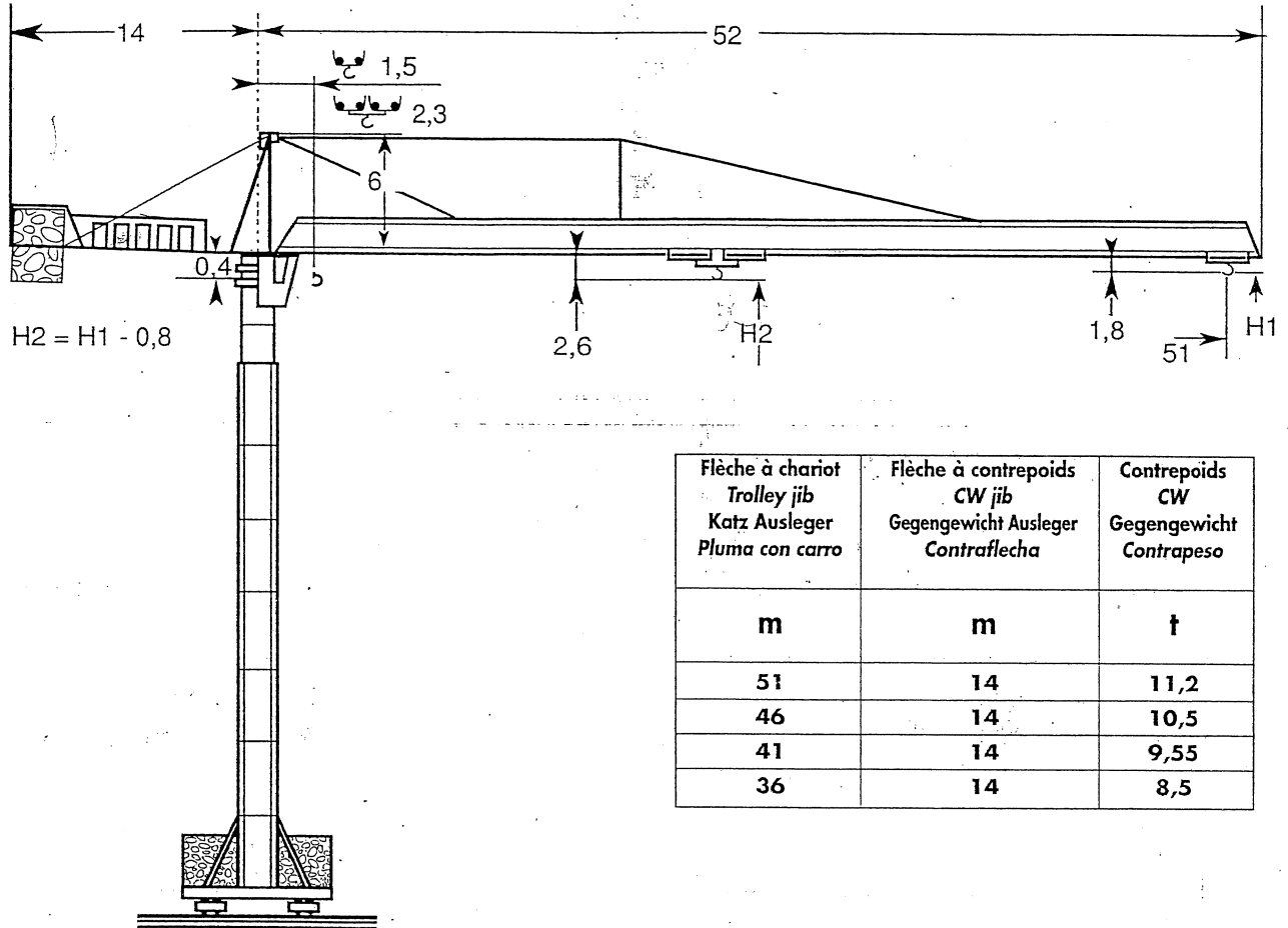
FLECHE - JIB - AUSLEGER - FLECHA 51 m
